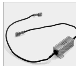
L4.73455.E Compensating resistance f. electronic hour counter Vorwiderstand f. elektr. Betriebsstundenzähler
