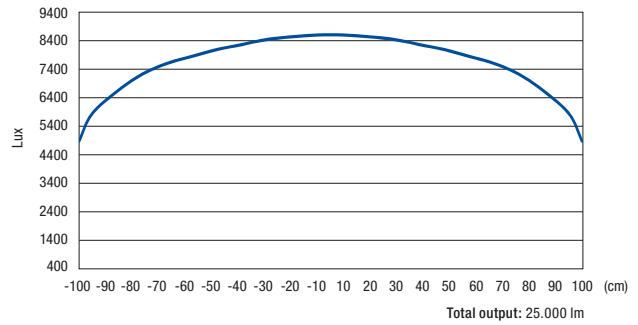
P12 Lichtverteilung
